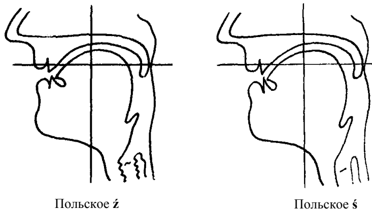
Рис. 67. Артикуляционные профили польских согласных ż и ś (Bał 1977: 70)
