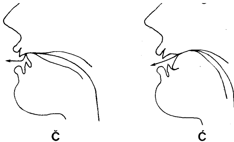
Рис. 38: Артикуляция согласного ʃ и tʃ (Škarić 1991: 131)
