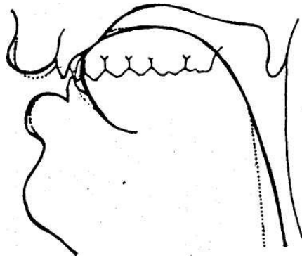
Рис. 37: Артикуляционные профили звуков ʃ и tʃ : сплошная линия — ʃ , пунктирная линия — tʃ (Miletić 1960: 41)
