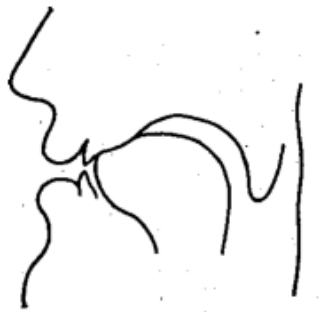
Рис. 58. Артикуляция серб.-хорв. ɲ (Popova 1986: 28)
