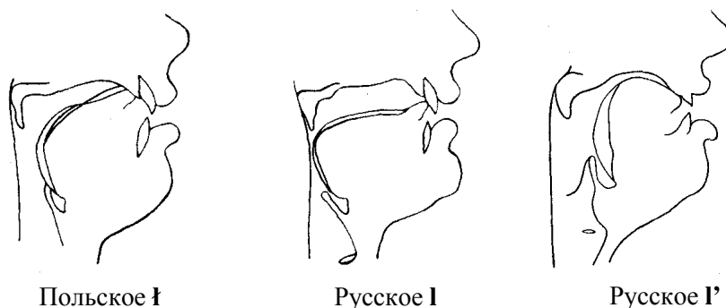
Рис. 65. Артикуляционные профили польского ɫ и русских согласных ɫ и ɫ' (Karolak/Wasilewska 1977: XXV)
