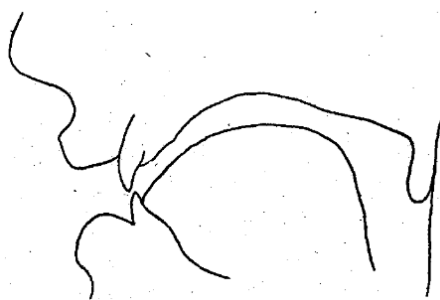
Рис. 26. Артикуляция сербохорватского гласного е (Jazić 1966: 26)
