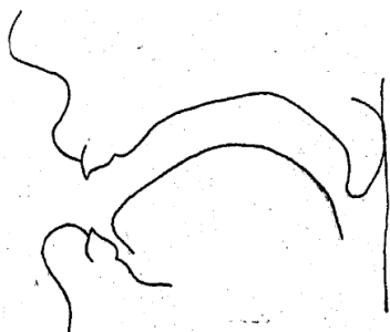
Рис. 25. Артикуляция русского открытого гласного е [ɔ] (Jazić 1966: 26)
