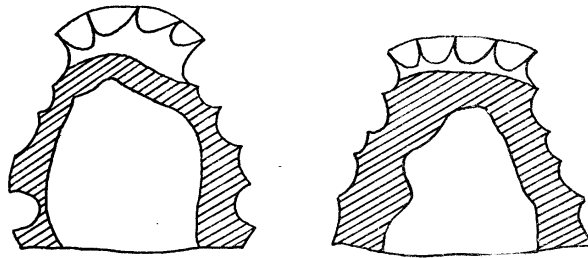
Рис. 62. Слева – палатограмма сербскохорватского \text{ʃ} в слово mūčī (по Милетичу).
