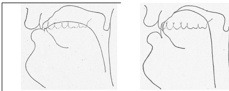
Рис. 43: Артикуляционные профили звуков I (слева) и Ī (справа) – Miletić 1960: 25, 32
